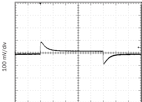
Load 50 - 100 - 50%, 50 Vin
