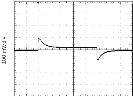
Load 50 - 100 - 50%, 28 Vin
